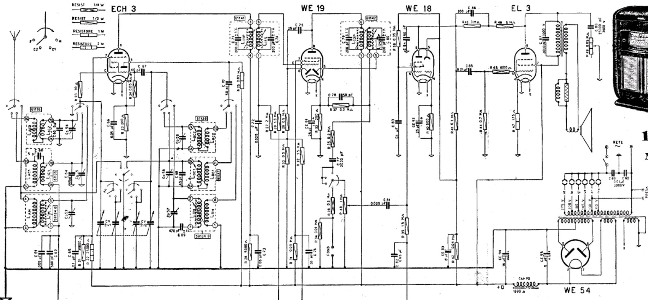
— LA VOCE DEL PADRONE. — Mod. MARCONI 1562. — Telaio 621. — Serie sintorapida. — Produzione 1941-1942. — Cinque valvole: ECH3, WE19, WE18, EL3, WE54. — Occhio magico WE18. — Tre gamme d'onda: onde medie 192 a 576 m; onde corte prime 24 a 53 m; onde corte seconde 14 a 24 m. — Media frequenza: 465 kHz. — Altoparlante medio esponenziale. — Alimentazione a corrente alternata da 100 a 275 volt. — Potenza d'uscita indistorta: 3 watt. — Consumo: 50 watt circa. — Peso: kg. 39 circa. — Dimensioni d'ingombro: cm. 40 x 60 x 90.
